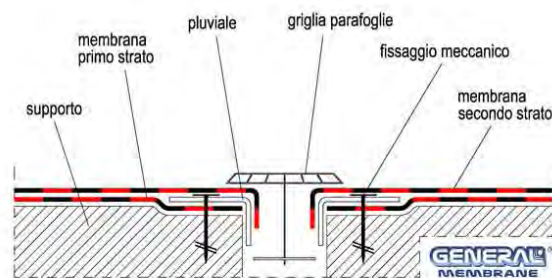
Fig. 11 – Scarico di un Pluviale
