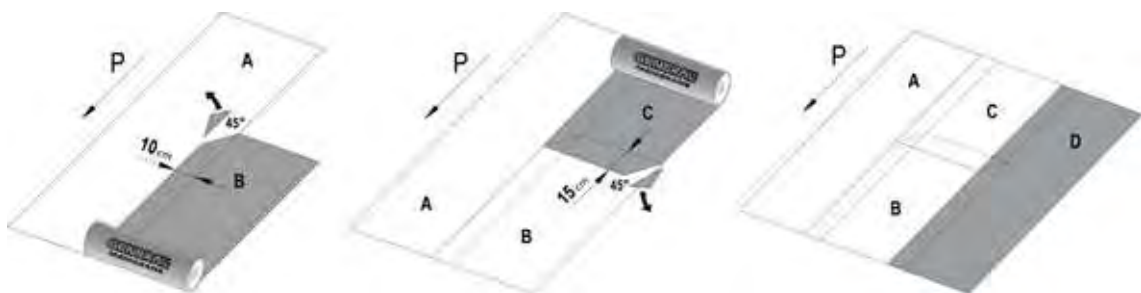
Fig.7 – posa in MONOSTRATO o PRIMO STRATO: posizionamento teli e esecuzione saldature sezione corrente (le lettere indicano la successione di posa dei fogli con indicazione delle misure delle sovrapposizioni laterali e di testa)
