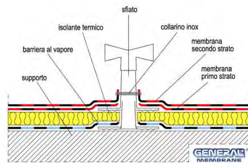
Fig. 19 - Sfiato su estradosso con stratigrafia coibentata
