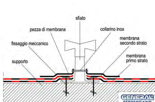
Fig. 18 - Sfiato/Areatore con fissaggio meccanico
