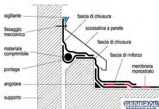
Fig. 29 – Giunto di dilatazione a parete
