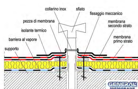
Fig. 21 - Sfiato doppio corpo collegato a ambienti interni
