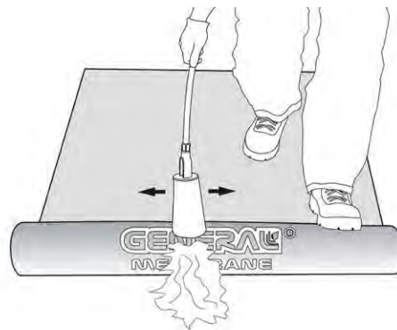
Fig. 1- Esempio di posa in totale aderenza mediante fiamma generata da bruciatore a gas propano
