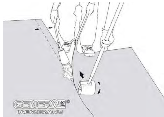
Fig 3 - Esempio di posa a secco in indipendenza, con sola saldatura delle giunzioni mediante fiamma generata da bruciatore a gas propano
