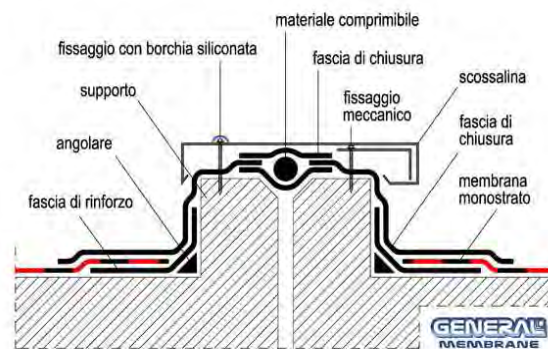
Fig. 28 – Giunto di dilatazione in rilievo
