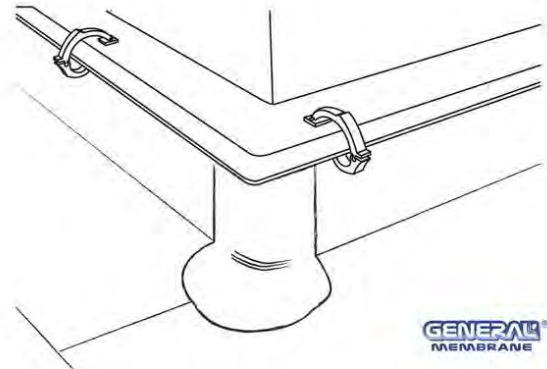
Fig. 25 – lucernaio: rinforzo dell'angolo
