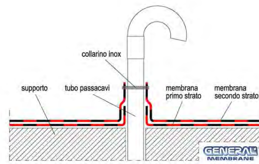
Fig. 23 - Tubo passante senza pezzo speciale
