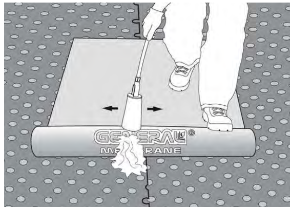
Fig.2 - Esempio di posa in semiaderenza mediante fiamma generata da bruciatore a gas propano (Membrana forata di base: PEGASUS SPOT non oggetto del presente Certificato)
