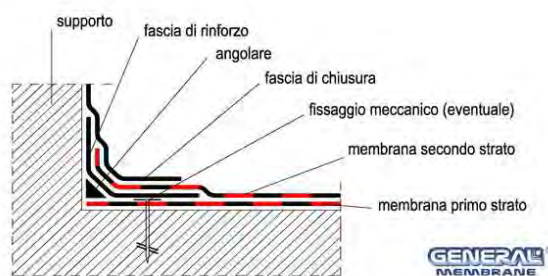
Fig. 15 - risvolto verticale doppio strato – Tipo 3
