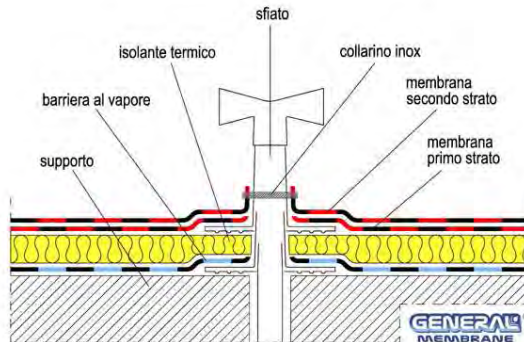
Fig. 20 - Sfiato doppio corpo collegato alla barriera vapore
