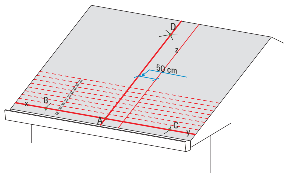
Fig. 1 - Trasarea acoperișului
